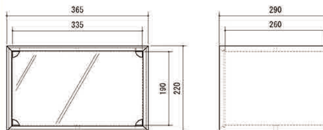
寸法図 (mm)
